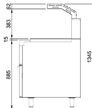
End Elevation
